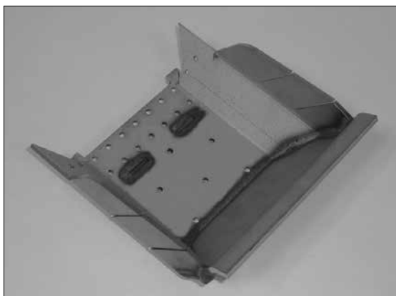
Камера сгорания горелки для пневмоочистка
