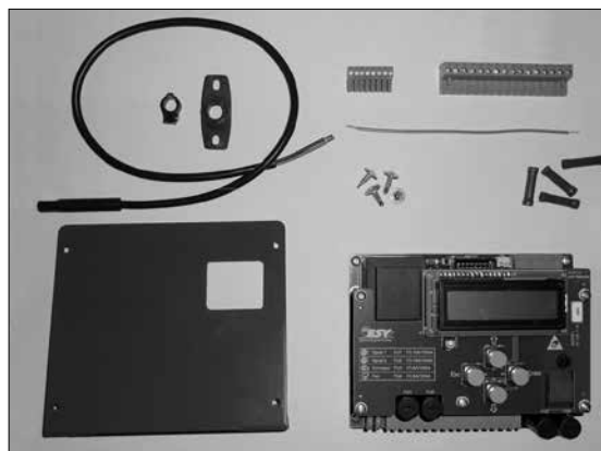
Комплект для перестройки на электронный модуль AC07X
